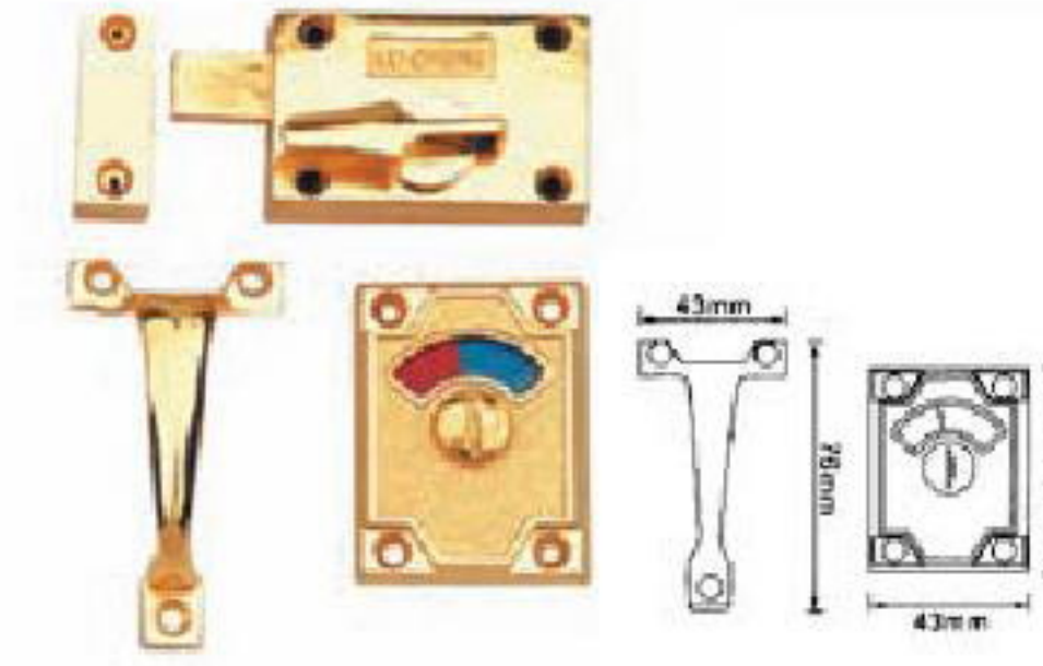
MODEL: G-6083 MATERIAL: ZINC ALLOY
