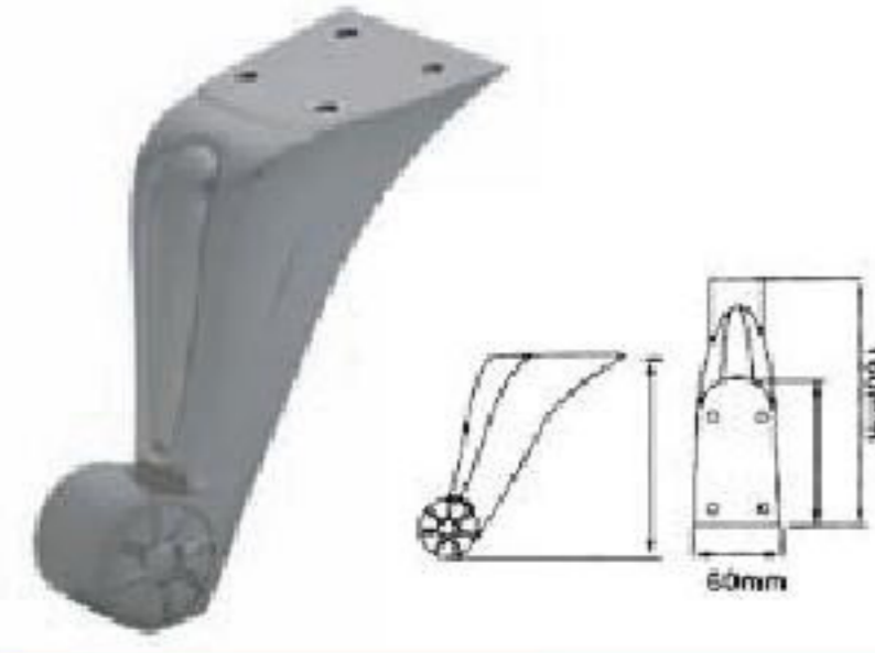
■ MODEL: G-6135 MATERIAL: ZINC ALLOY
