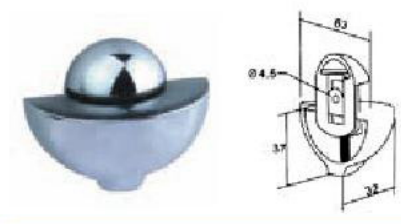
■ MODEL: G-6200 MATERIAL: ZINC ALLOY
