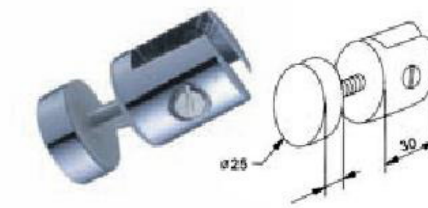
■ MODEL: G-6198 MATERIAL: ZINC ALLOY
