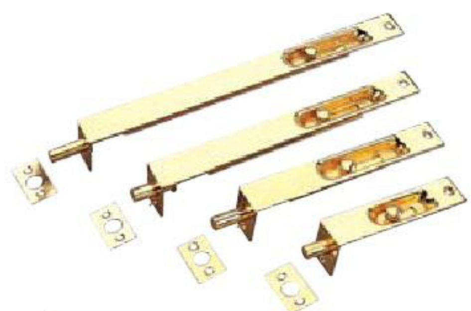
Number C710 Length 10" 8" 6" 4" Width 23mm 23mm 23mm 23mm
