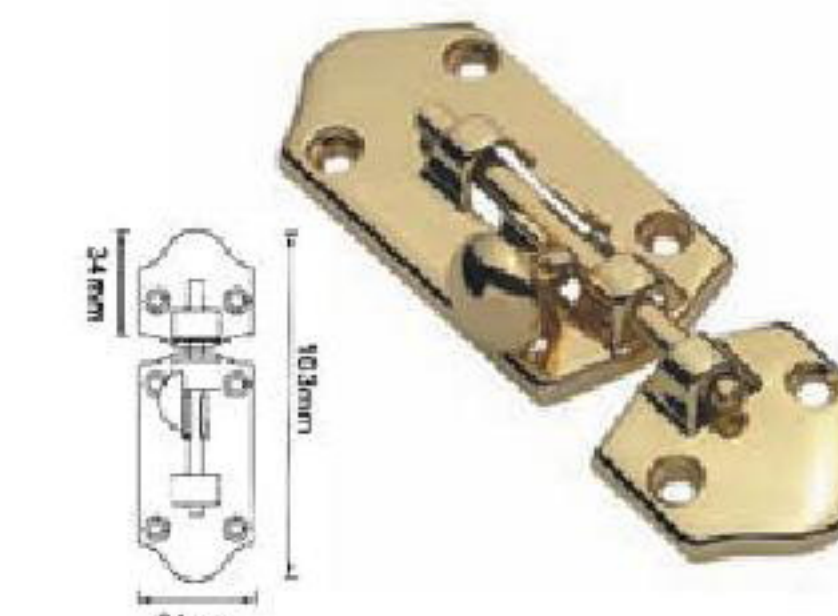
MODEL: G-6093 MATERIAL: ZINC ALLOY
