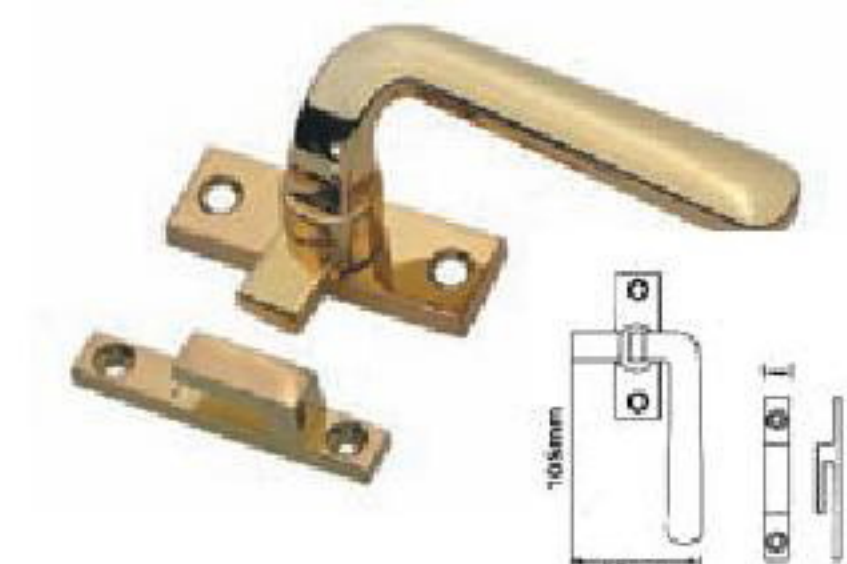
MODEL: G-6086 MATERIAL: ZINC ALLOY
